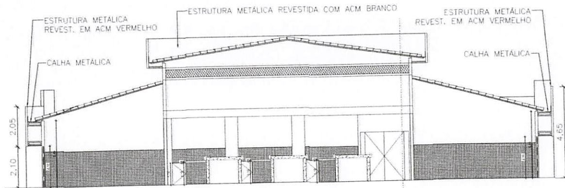
01 CORTE A
